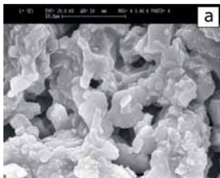
Figura 8. Microfotografías por MEB de minerales neoformados por la alteración de edificios históricos. (a) Cristales de yeso, \text{CaSO}_4 \cdot 2\text{H}_2\text{O} ; (b) cristales de halita, \text{NaCl} ; (c) esferas de fosfato de calcio. Estos minerales sugieren que los principales elementos indicadores de alteración son azufre, cloro y fósforo.
