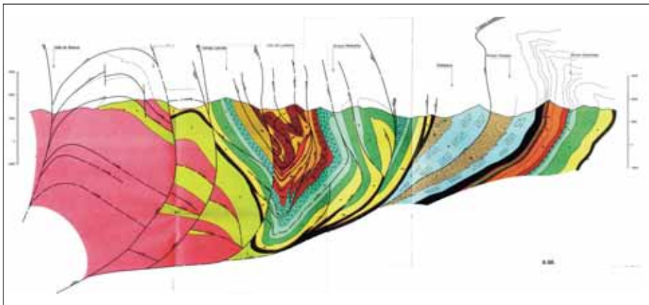
Figura 6. Corte geológico.
